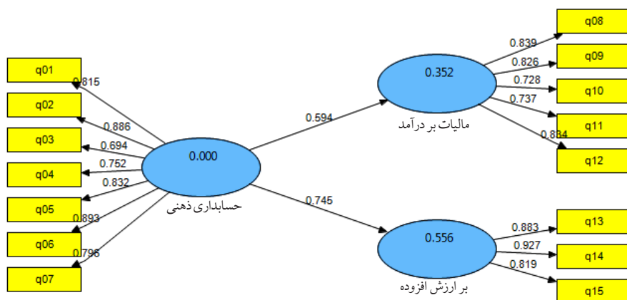
نمودار ۱. مدل در حالت ضرایب استاندارد
