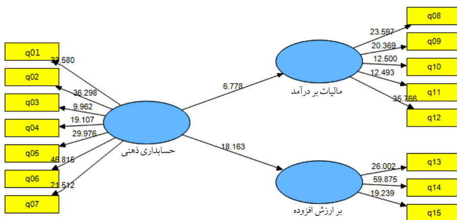
نمودار ۲. آماره t مدل در حالت ضرایب استاندارد
